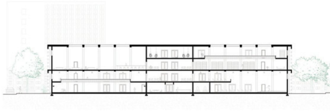
Longitudinal Section | 1/16" = 1'-0"
